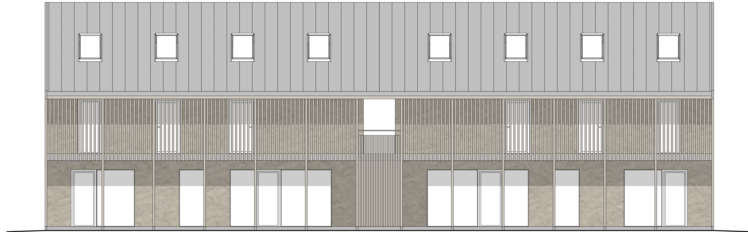
POHLED V, DO ZAHRAD
