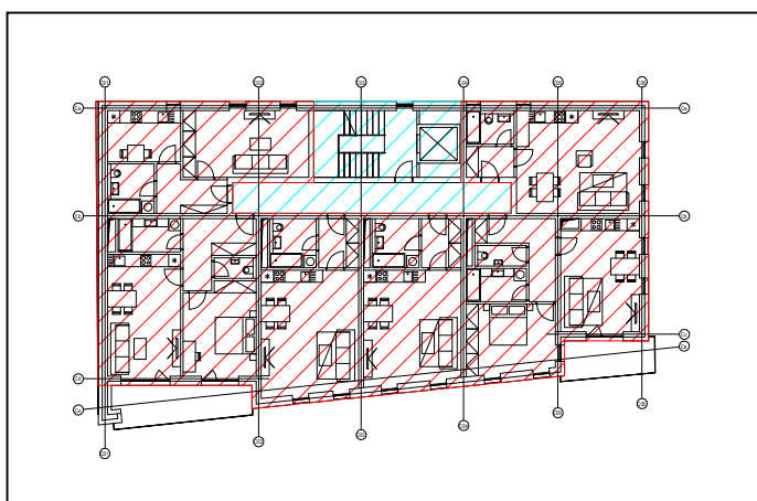
Obr. 4 – půdorys 4NP
