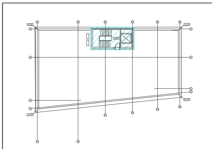
Obr. 7 – půdorys střechy
