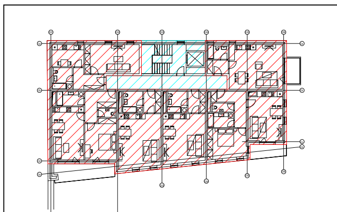
Obr. 3 – půdorys 3NP
