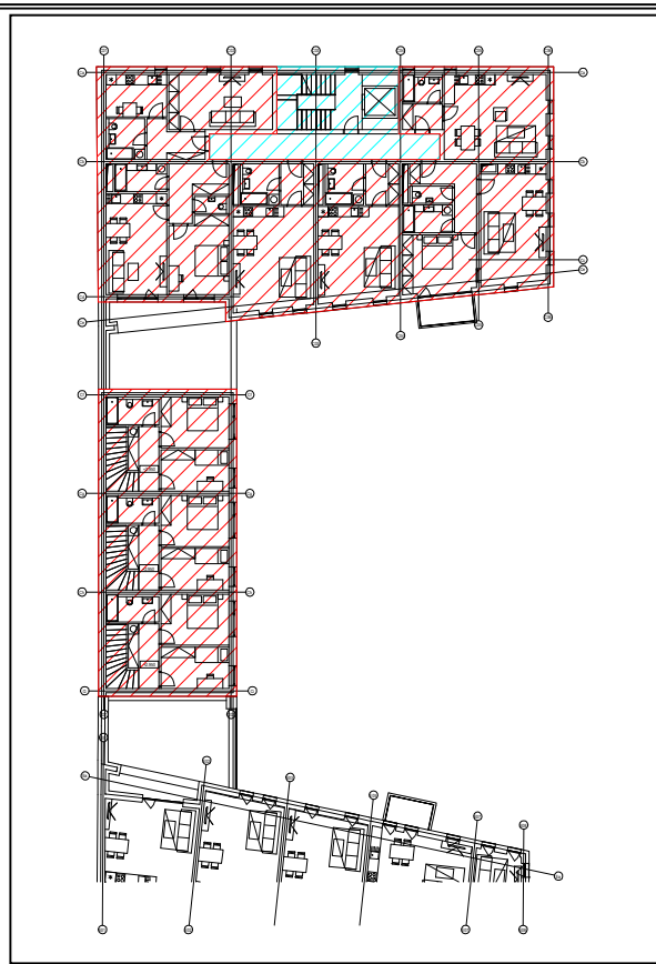
Obr. 2 – půdorys 2NP
