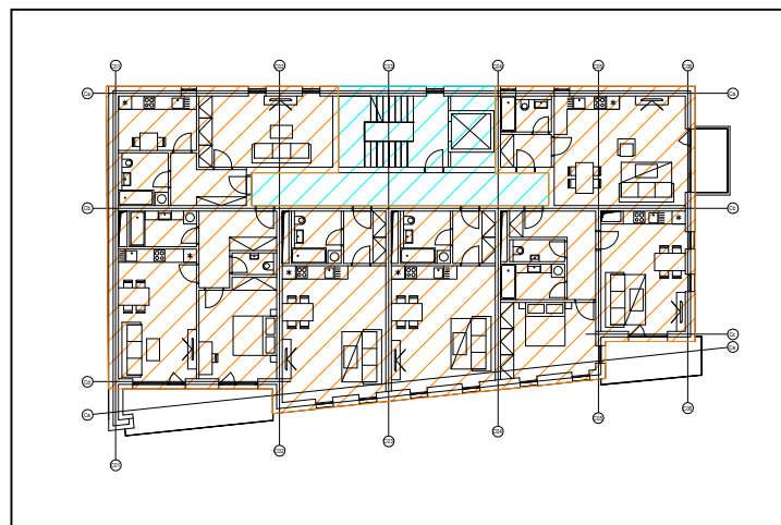
Obr. 6 – půdorys 6NP
